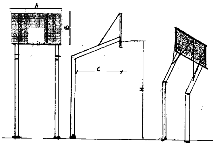
Rys. 2 Zestaw do koszykówki zewnętrznej z tablicą gretingową
