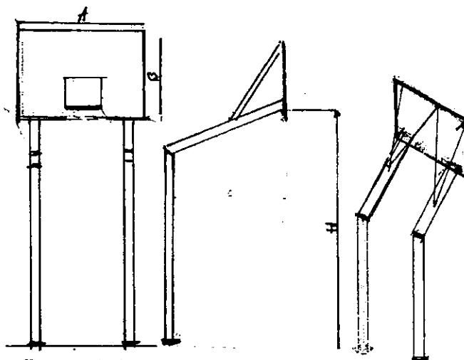
Rys.1 Zestaw do koszykówki zewnętrznej z tablicą epoksydową
