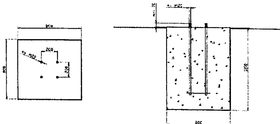
Rys 3 Zalecenia do wykonania stopy fundamentowej
