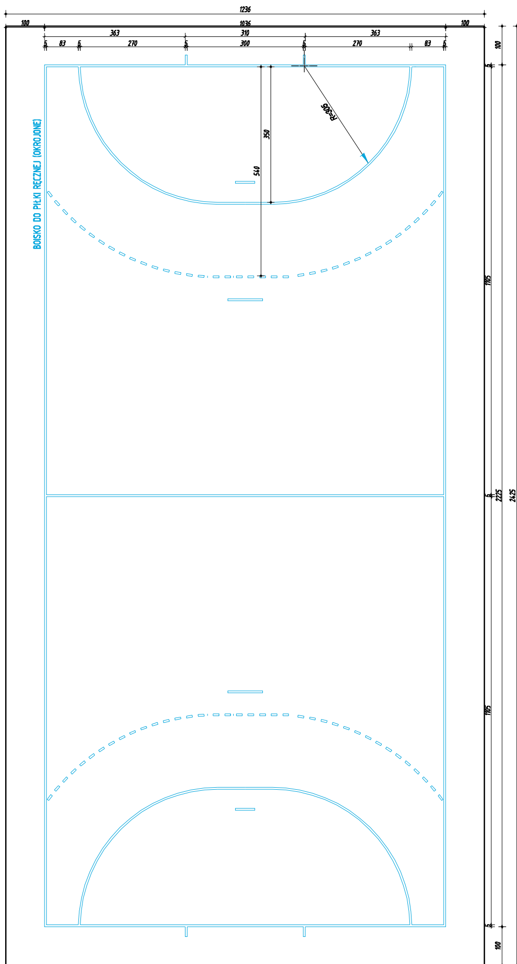
OBRYŚ SALI GIMNASTYCZNEJ
