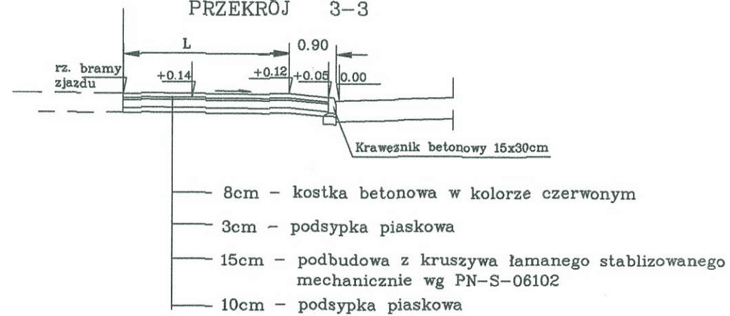
PRZEKRÓJ 3-3
