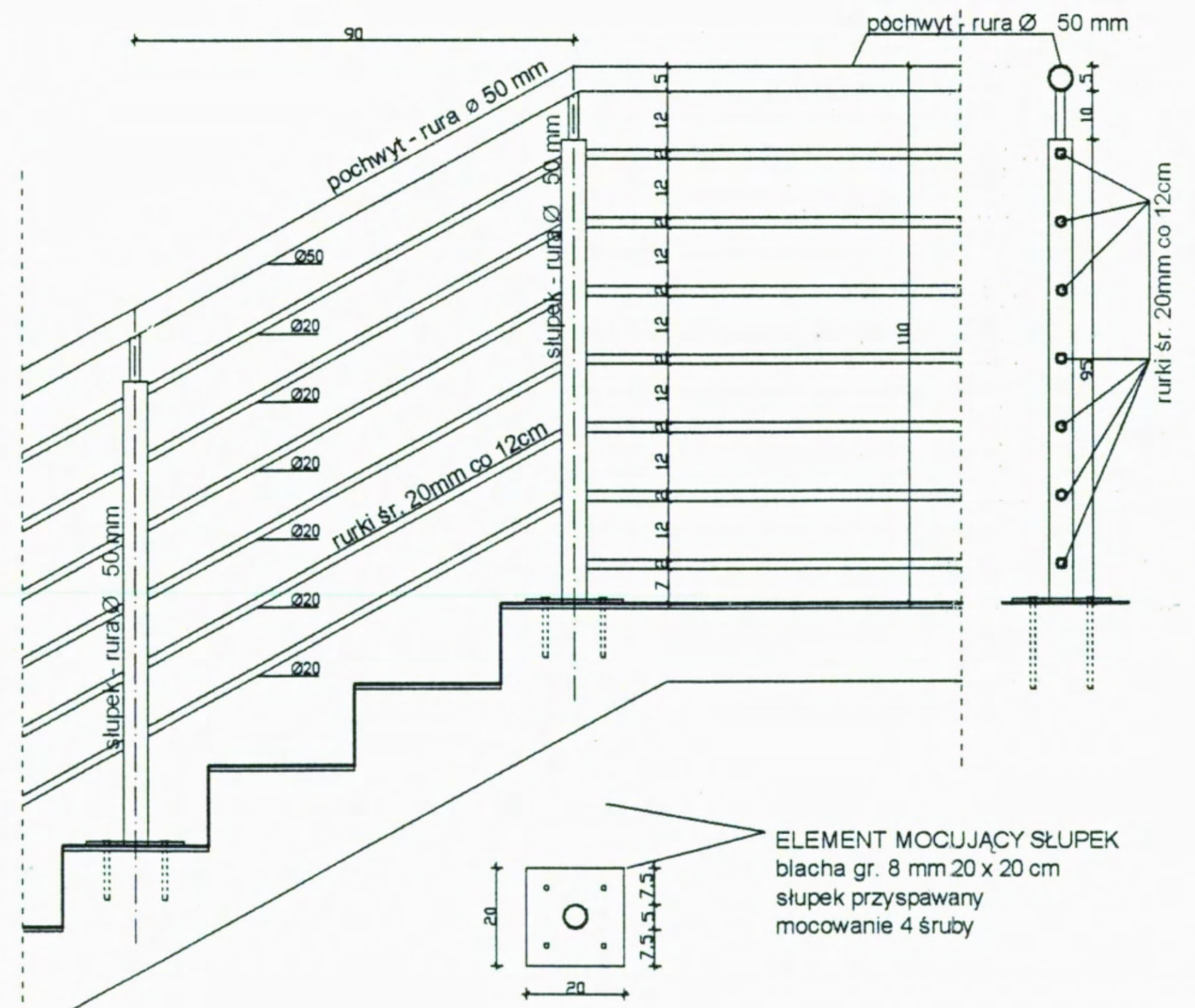
BALUSTRADA B-2 prześło na schodach SKALA 1:20
