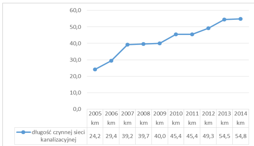
Wykres 19 Długość czynnej sieci rozdzielczej kanalizacyjnej w Gminie Halinów w latach 2005-2014 [km]
