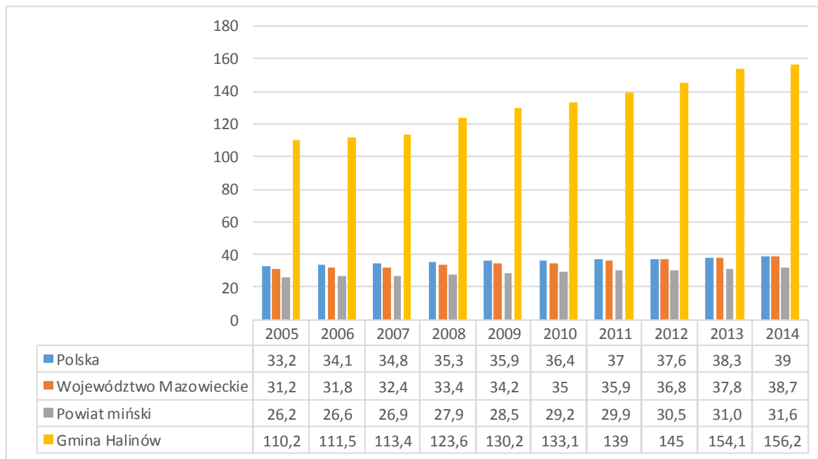
Wykres 22 Wskaźnik rozdzielczej sieci gazowej na 100 km w gminie Halinów na tle danych dla powiatu mińskiego, województwa mazowieckiego i Polski w latach 2005-2014
