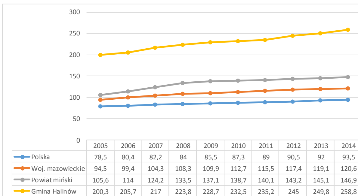
Wykres 18 Długość sieci rozdzielczej wodociągowej na 100 km w Gminie Halinów na tle wskaźników przyjętych dla powiatu mińskiego, województwa mazowieckiego i Polski w latach 2005-2014 [km]
